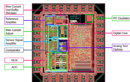
Bild 4: Chip-Plot mit den Bezeichnungen der Funktionsblöcke
