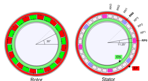
Bild 3: Codescheiben des Rotationsencoders
