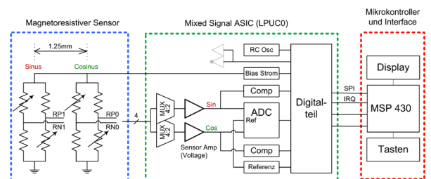
Bild 2: Blockdiagramm der magnetoresistiven Längenmessung
