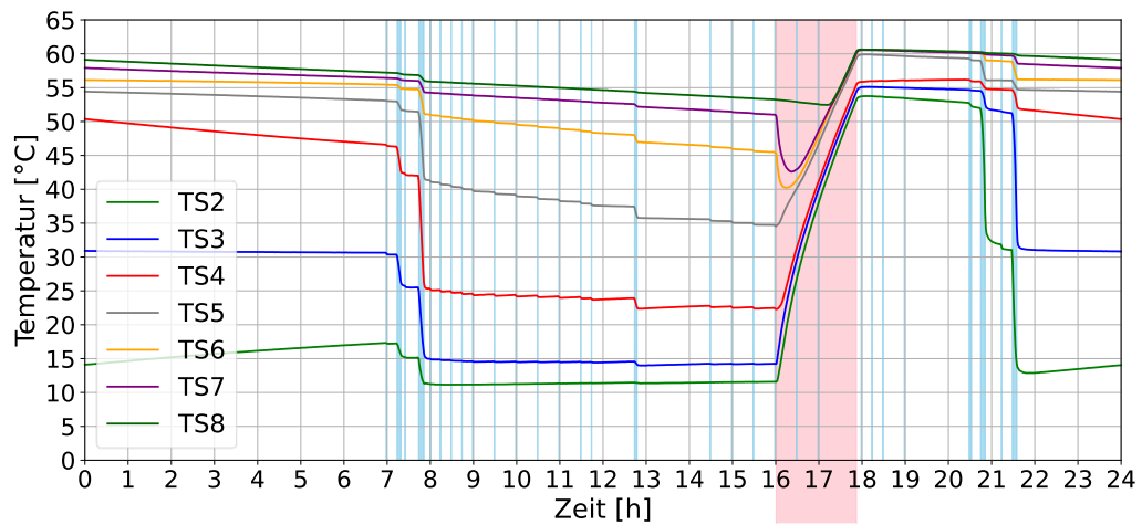
Abbildung 12 Speicher G, Speichertemperaturen TS aus Messdaten über die Zeit, blauer Hintergrund markiert eine Entladung und roter Hintergrund markiert eine Beladung
