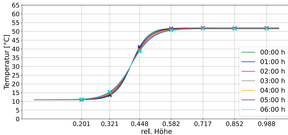
Abbildung 35 Standby Speicher F mit \%_{\Delta T, SIA} = 5.52 \cdot 10^{-5} , T_{min,initial} = 10.9 \text{ }^\circ\text{C} , T_{max,initial} = 52 \text{ }^\circ\text{C} , b = 0.43
