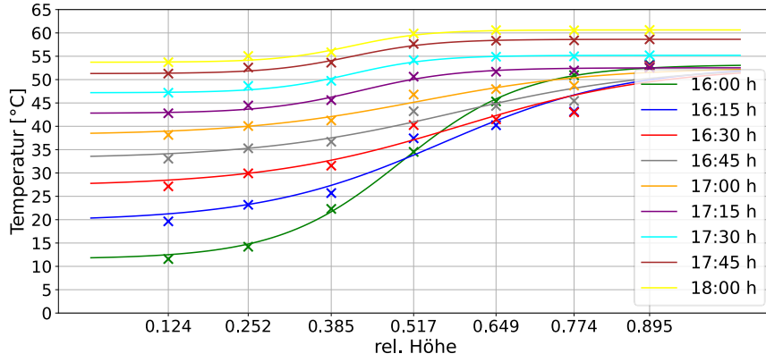
Abbildung 80 Beladung, Speicher G
