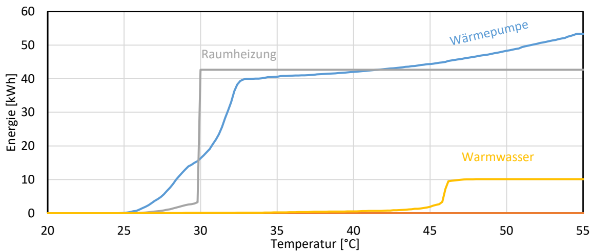
Abbildung 63: Energie-Temperatur Diagramm aus Test 1
