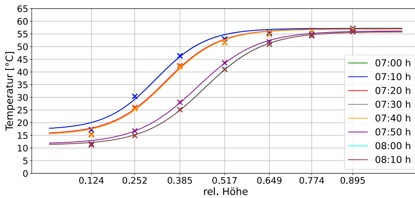
Abbildung 78 Entladung am Morgen, Speicher G
