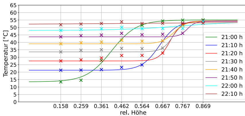
Abbildung 86 Beladung am Abend, Speicher H
