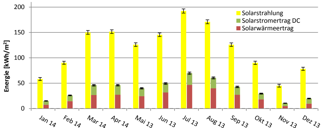
Abbildung 47: Monatswerte für die Solarstrahlung und der Erträge der PVT-Anlage auf dem SPF-Testdach.
