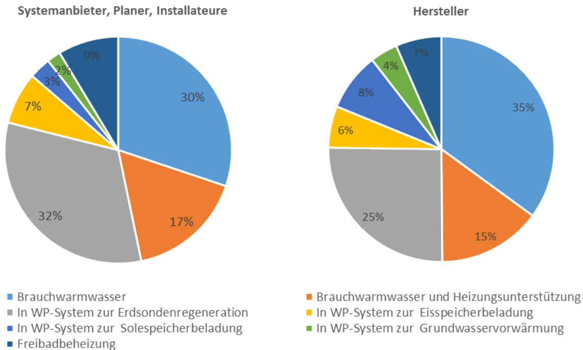
Abbildung 58: Verteilung der Anzahl von PVT-Anlagen in Betrieb in der Schweiz nach Systemeinsbindung laut Angaben der Systemanbieter, Planer und Installateure sowie der Hersteller
