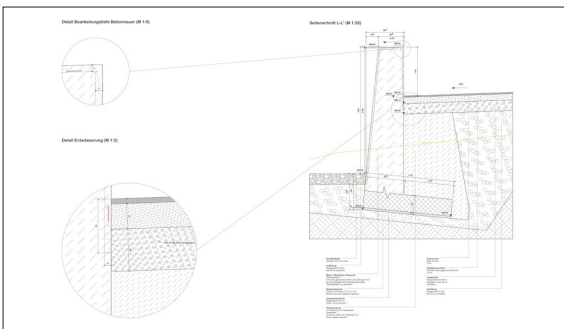
Ausführungsplanung – Schnitt Mauer «Schotterbeton»
