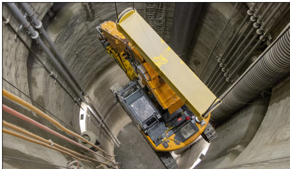
Der knapp 50 tonnenschwere Tunnelbagger wird durch den Schacht in die Kaverne gehoben Eigene Darstellung
