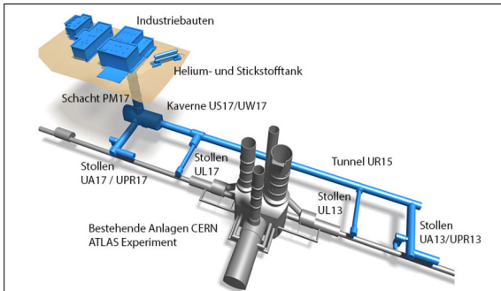
Die neuen Infrastrukturanlagen (blau) am Point 1. Neben den Untertagbauten entstehen an der Oberfläche Industriebauten Credit: CERN
