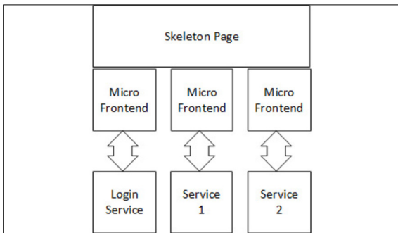
Micro-Frontend HTML Frontend-Architektur
