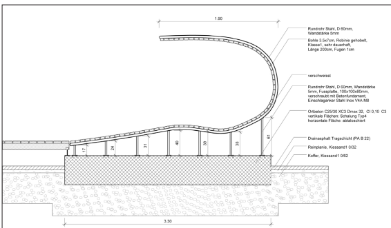
Schnitt: Liegeelement
