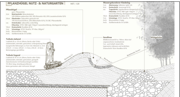
Detailschnitt Nutz- & Naturgarten Eigene Darstellung
